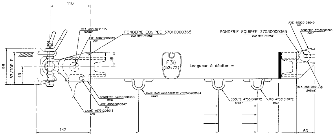
VIT DE MULET COMPLET 34511770C05 COMPLETE GOOSENECK
