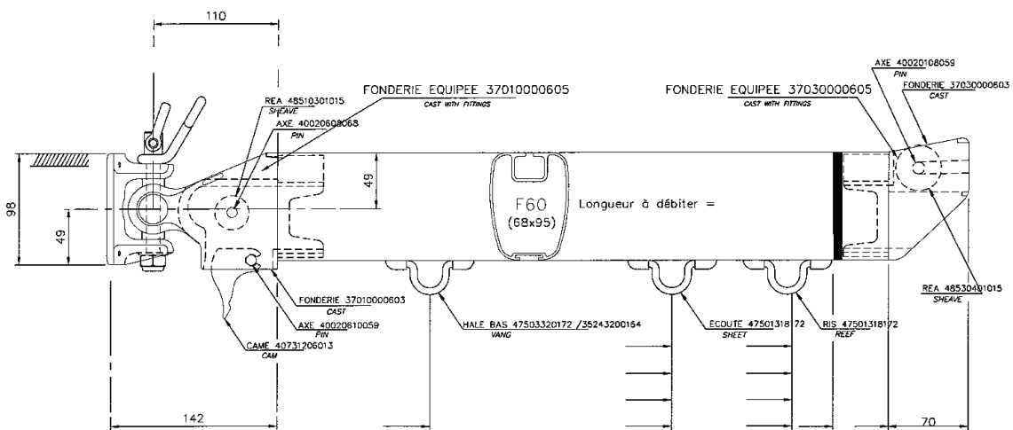
Vit de Mulet complet 34511770C15 COMPLETE GOOSENECK
