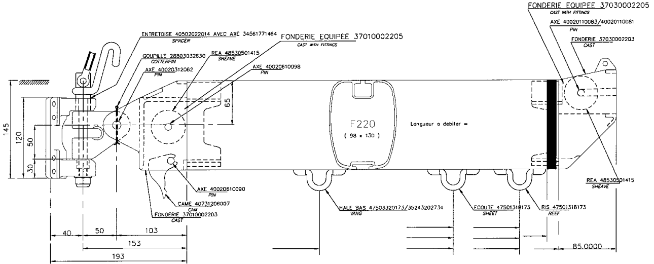
VIT DE MULET COMPLET 34511770C25 COMPLETE GOOSENECK
