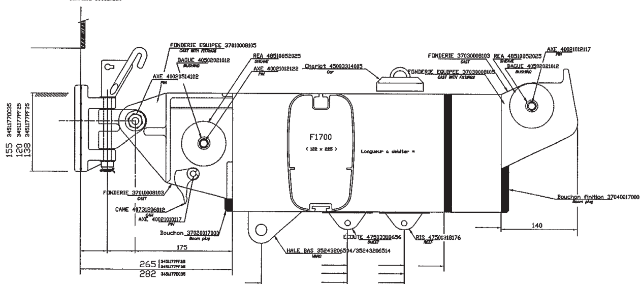
VIT DE MULET COMPLET 3451177PF25 / 3451177PF35 / 3451177DC35 COMPLETE GOOSENECK
